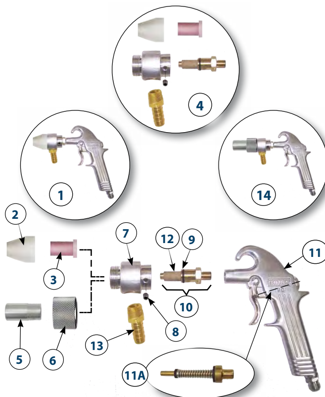
PISTOLET G15, LISTE DES PIÈCES
