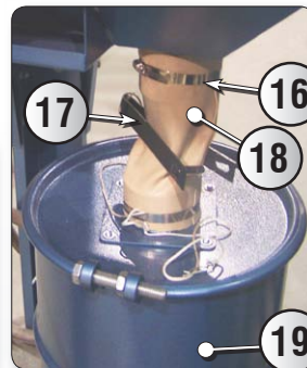
Trappe de vidange
