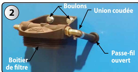
Connexion du boîtier de filtre
