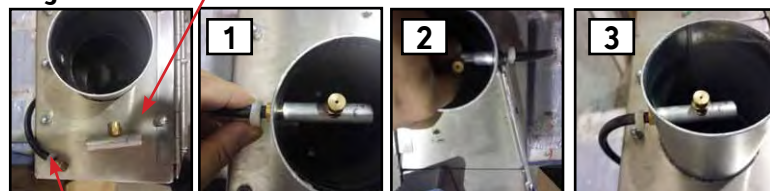
Tuyau d'air
